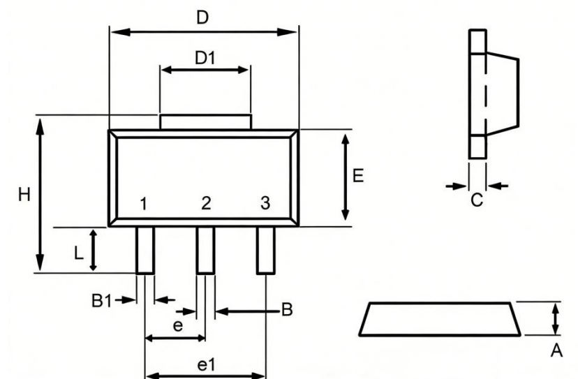
SOT-89
